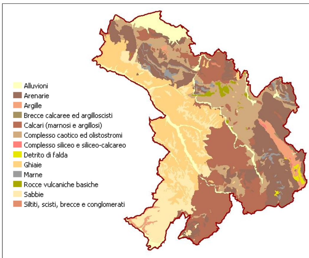
Fig. 6 Inquadramento geologico del territorio
