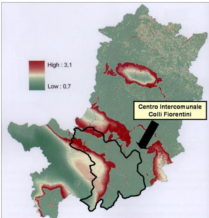
Fig. 9 Pericolosità sismica (INGV, 2006) e classificazione sismica dei comuni (Regione Toscana, 2014)
